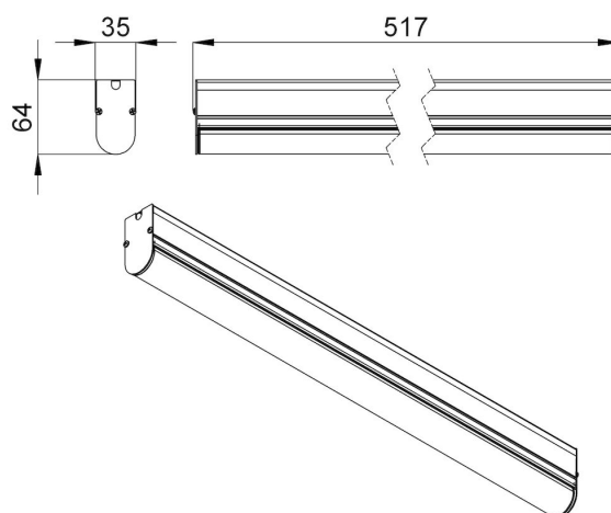
Габаритный чертеж
