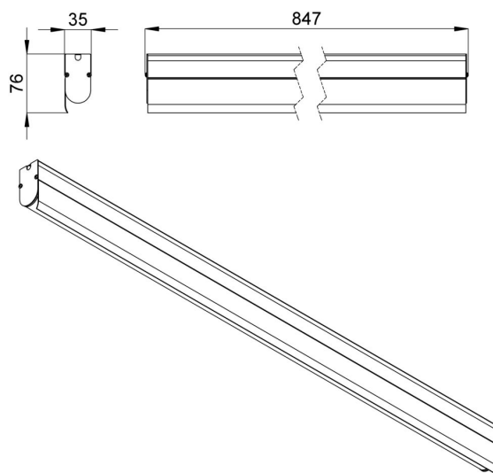
Габаритный чертеж
