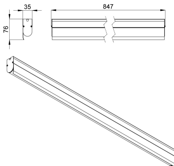
Габаритный чертеж
