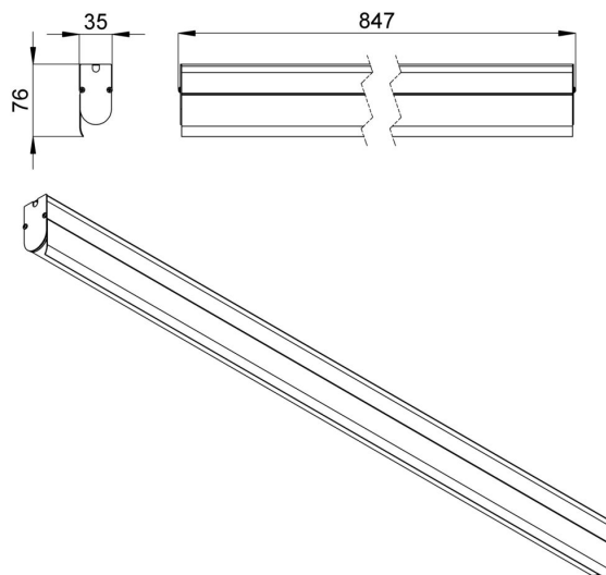
Габаритный чертеж
