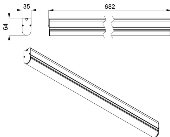
Габаритный чертеж
