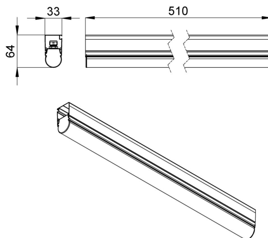
Габаритный чертеж
