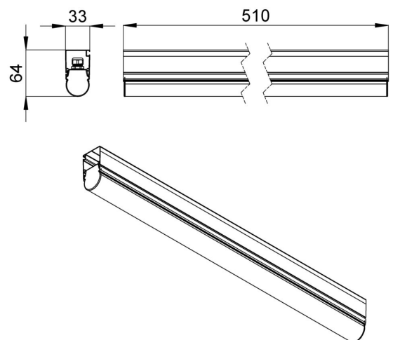
Габаритный чертеж
