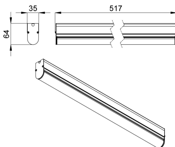
Габаритный чертеж
