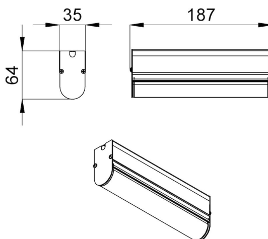
Габаритный чертеж
