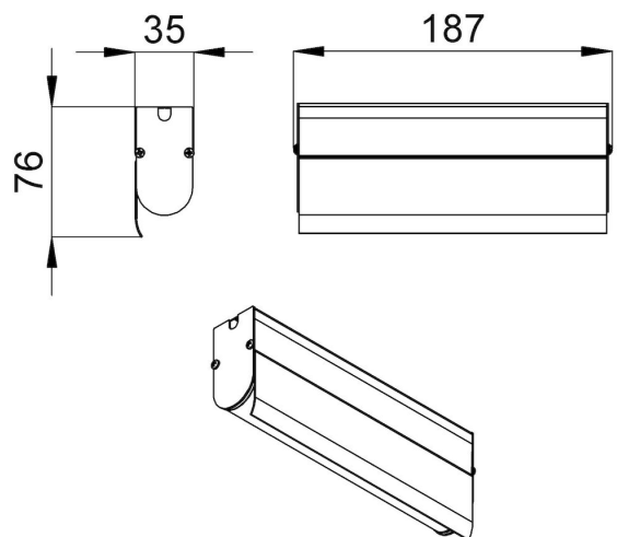
Габаритный чертеж
