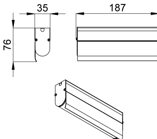
Габаритный чертеж
