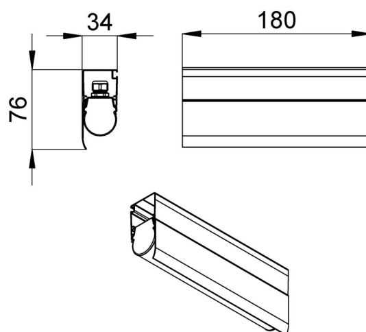
Габаритный чертеж
