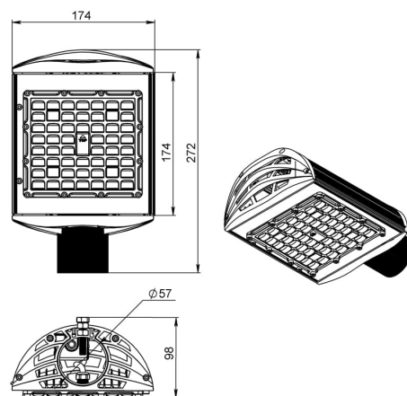
Габаритный чертеж
