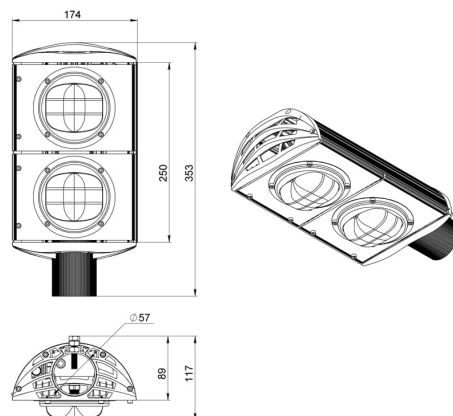
Габаритный чертеж
