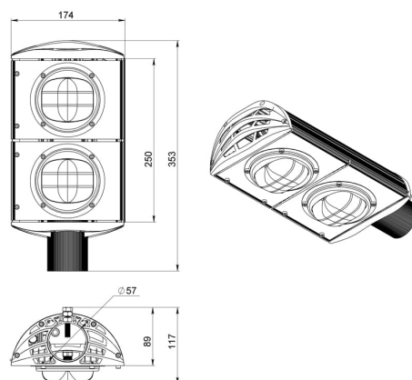
Габаритный чертеж
