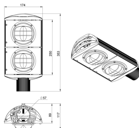
Габаритный чертеж
