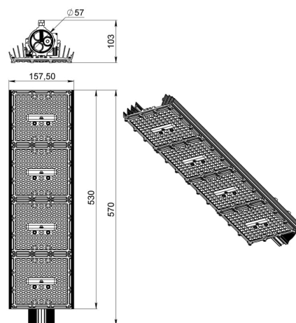
Габаритный чертеж
