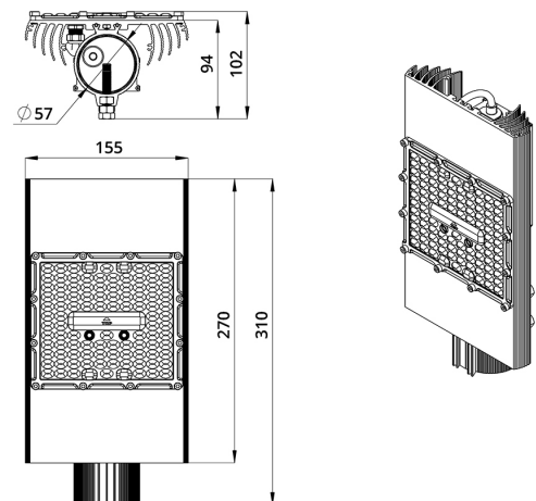
Габаритный чертеж
