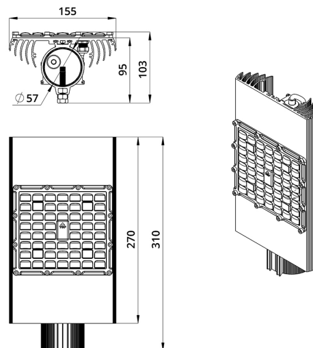
Габаритный чертеж
