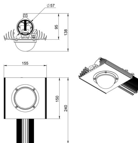
Габаритный чертеж
