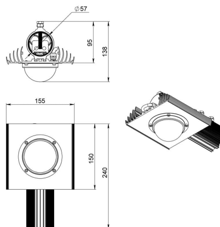
Габаритный чертеж
