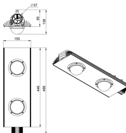
Габаритный чертеж
