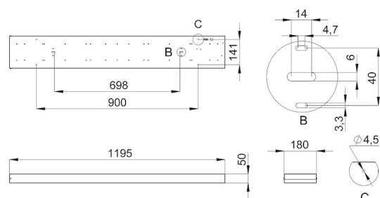
Монтаж светильника
