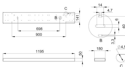
Монтаж светильника
