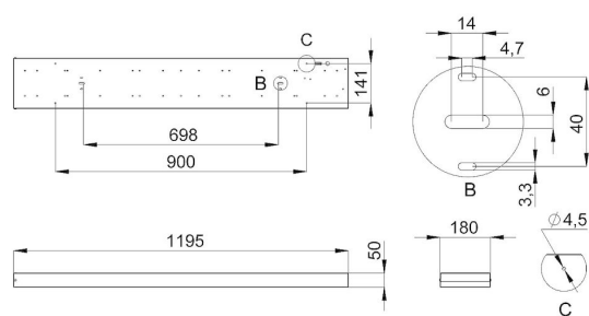
Монтаж светильника
