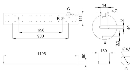
Монтаж светильника
