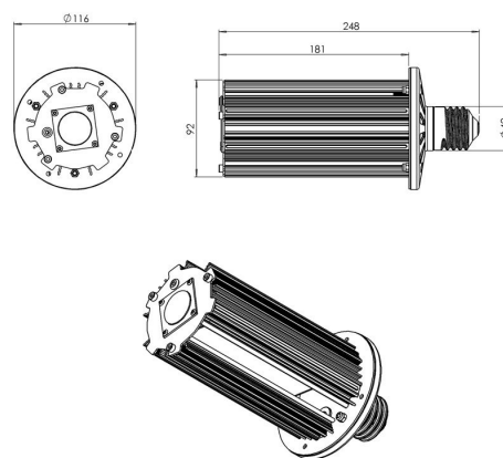
Габаритный чертеж
