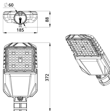
Габаритный чертеж
