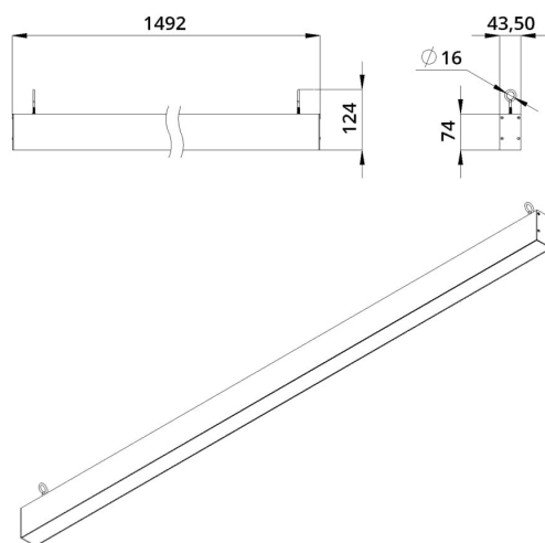
Габаритный чертеж
