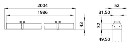
Габаритный чертеж
