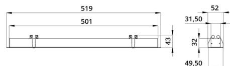
Габаритный чертеж
