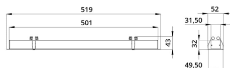
Габаритный чертеж
