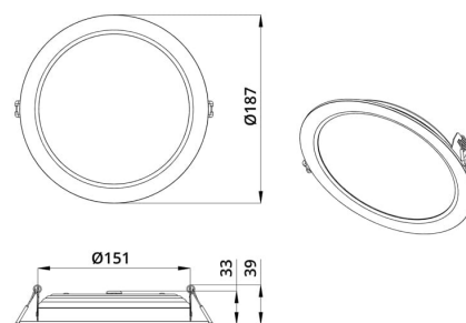
Монтаж светильника
