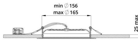
Монтаж светильника
