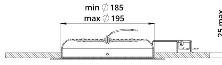
Монтаж светильника
