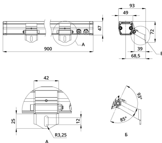
Габаритный чертеж
