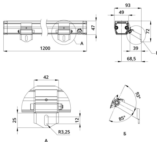
Габаритный чертеж
