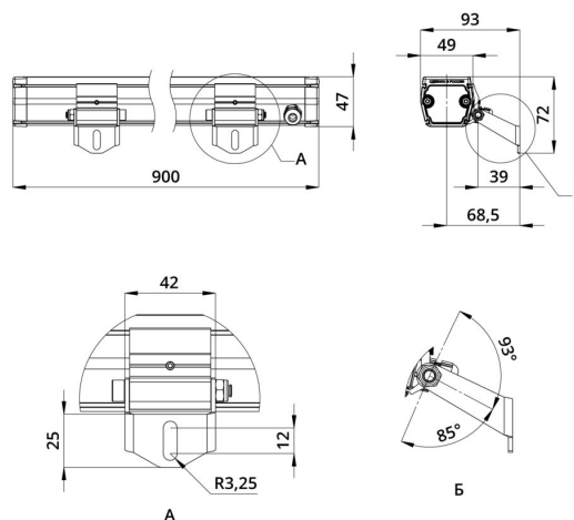
Габаритный чертеж
