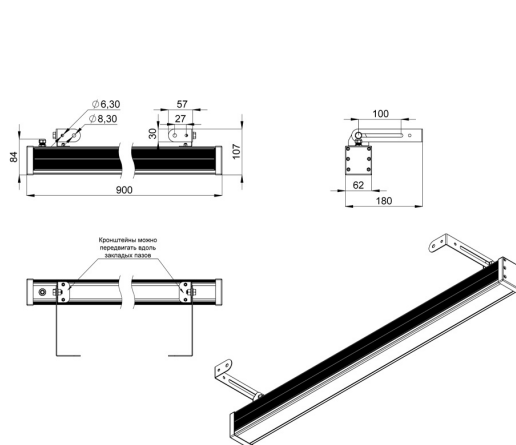
Габаритный чертеж
