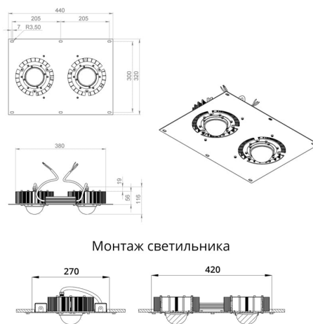
Габаритный чертеж
