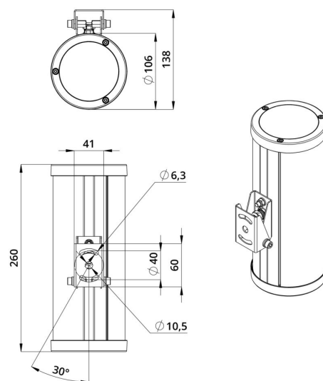
Габаритный чертеж
