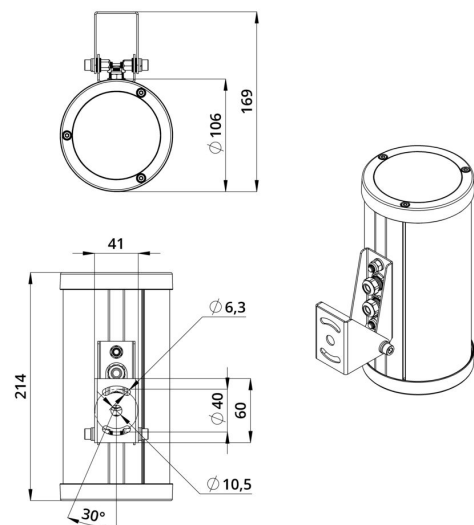
Габаритный чертеж
