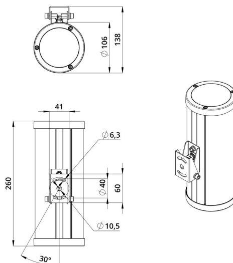
Габаритный чертеж
