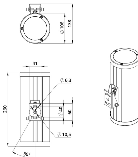
Габаритный чертеж
