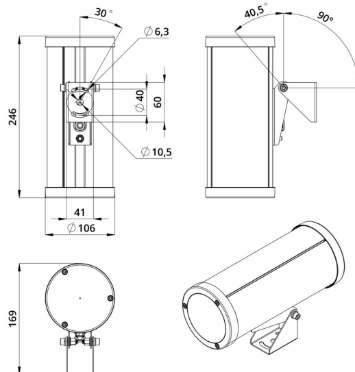
Габаритный чертеж
