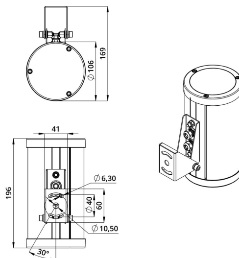
Габаритный чертеж
