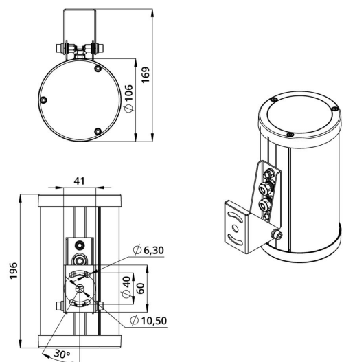
Габаритный чертеж
