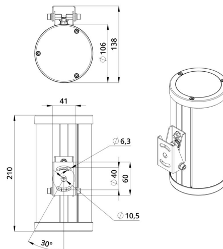
Габаритный чертеж
