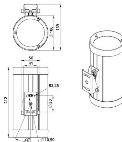
Габаритный чертеж
