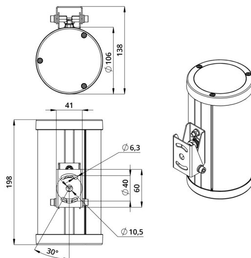
Габаритный чертеж
