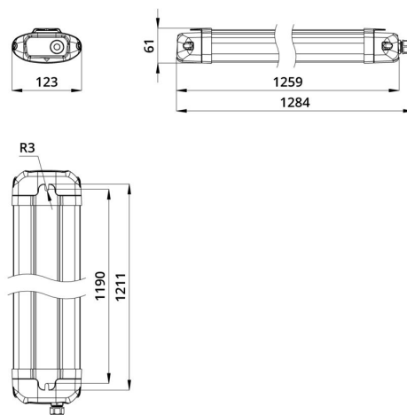
Габаритный чертеж
